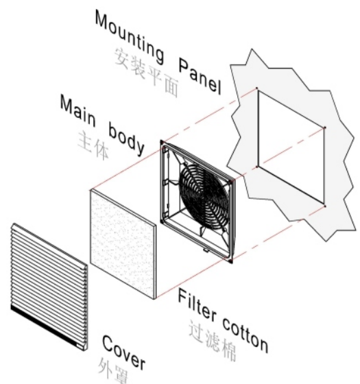
Mounting Method 安裝方法
