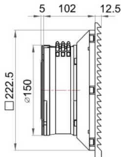
Fan & Filter 風扇及過濾器 M9804.230
