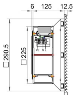
Fan & Filter 風扇及過濾器 M9805.230
