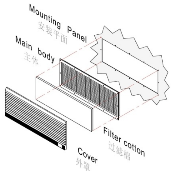
Mounting Method 安装方法
