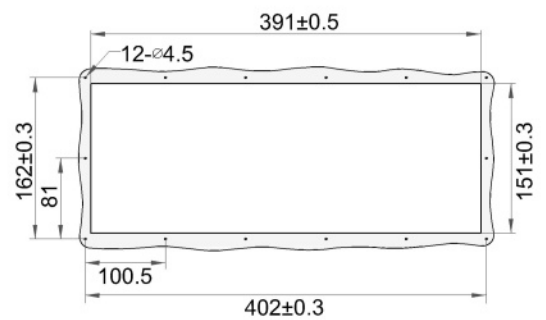
Mounting Method 安装方法
