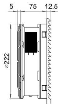
Fan & Filter 风扇及过滤器 M805.230
