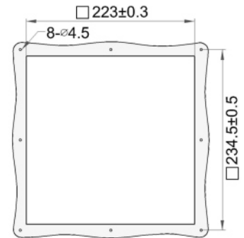
Mounting profile 安装剖面 M805
