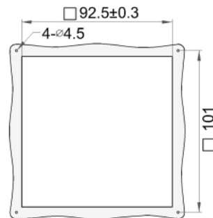
Mounting profile 安装剖面 M802
