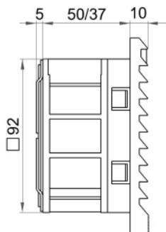
Fan & Filter 风扇及过滤器 M802.230
