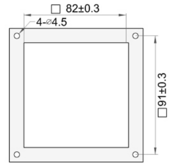
Mounting profile 安装剖面 M801
