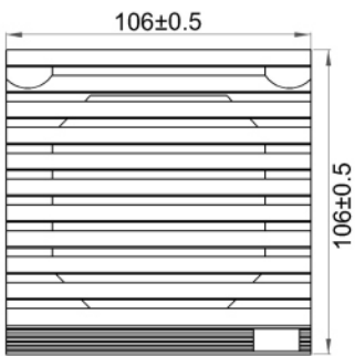
Fan Filter 风扇过滤器 M801
