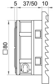
Fan & Filter 风扇及过滤器 M801.230
