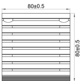
Fan Filter 風扇過濾器 M800
