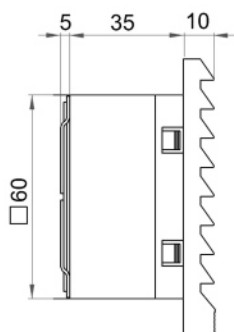
Fan & Filter 風扇及過濾器 M800.230
