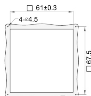
Mounting profile 安裝剖面 M800
